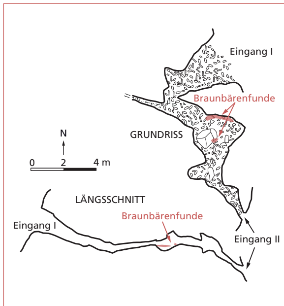
Abb. 2: Pläne der Sommerberghöhle I und Lage der Braunbärenfunde.
